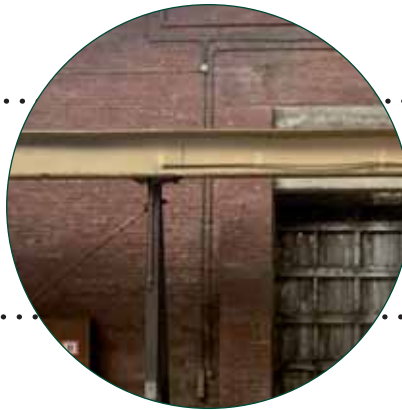
demontage herbruikbare delen stalen kraanbaan
