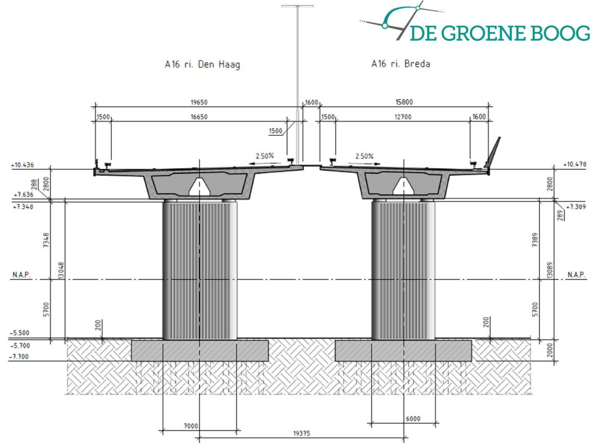
Dwarsdoorsnede brugdekken
